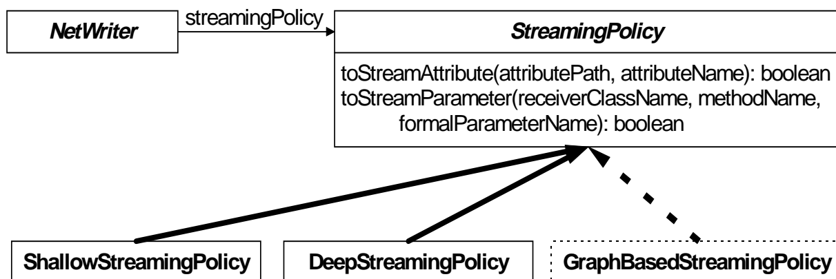
Abb. 6.1: Zusammenspiel NetWriter - StreamingPolicy
