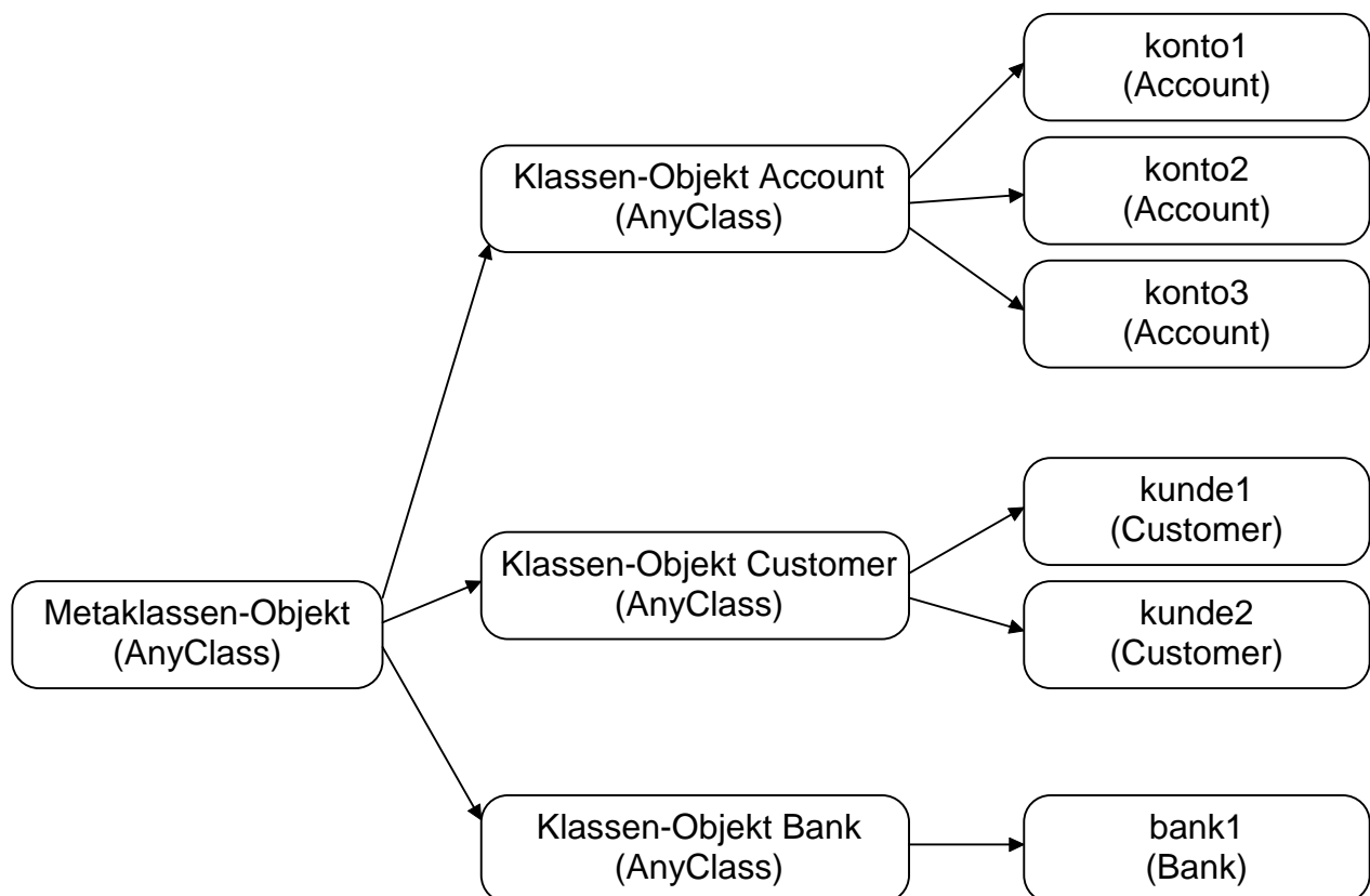
Abb. 3.2: Objektdiagramm der Metainformationen im VROOM System anhand eines Beispiels
