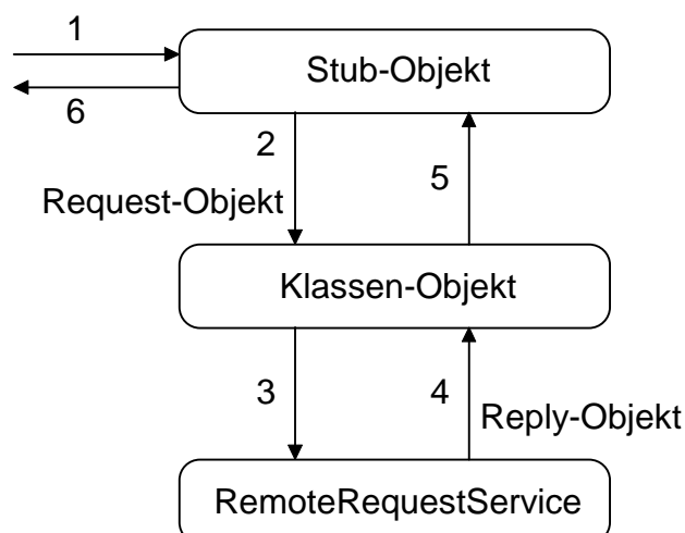
Abb. 7.2: Ferner Methodenaufruf
